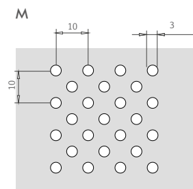
Para paso 300 Área perforada: diagonal Distancia entre ejes: 10x10 mm Superficie perforada: 14% aprox.
