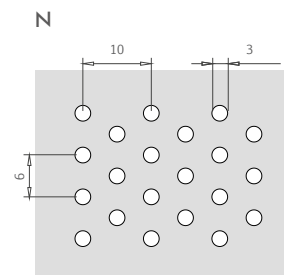
Par pas: 100 - 150 - 200 Zone perforée: diagonale Empattement: 10x6 mm Surface perforée: 23% approx.
