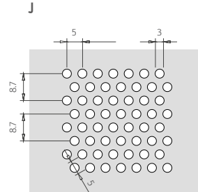
Par pas: 3 mm Zone perforée: diagonale Empattement: 5x8,7 mm Surface perforée: 32% approx.
