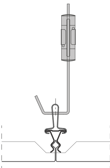
Sezione C -C'
