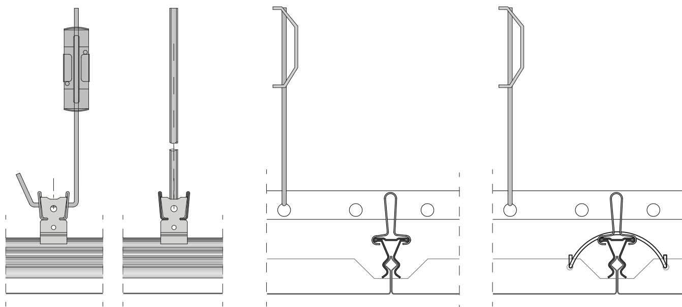
Sospensione con pendino
