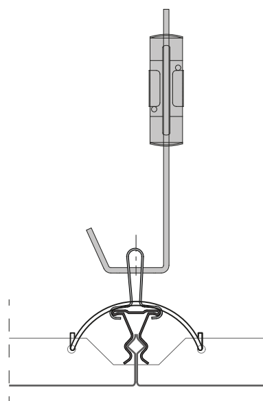
Sezione C -C' con molla antisganciamento
