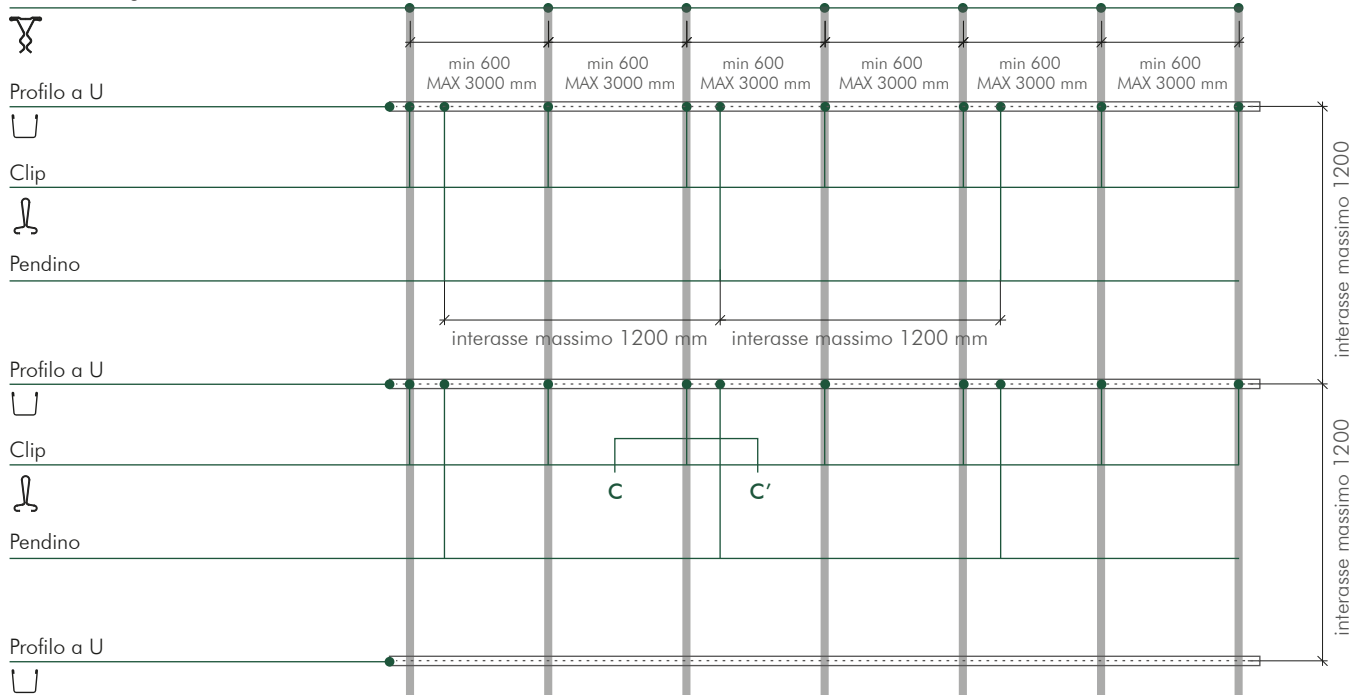
Profilo a triangolo + Giunto
