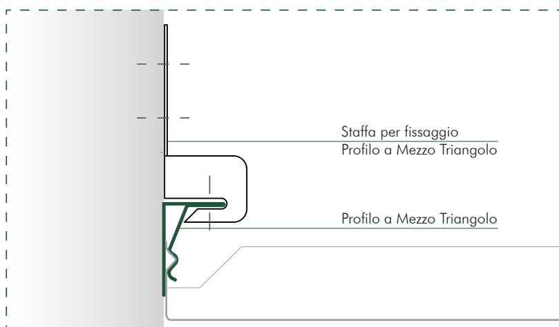
Profilo a Mezzo Triangolo_L 4000 mm
