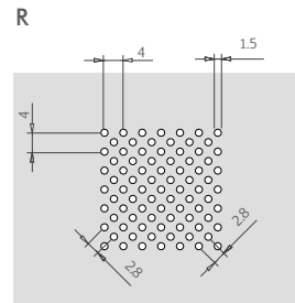
MICRO PERFORATION Diametro: 1.5 mm Area Perforata: diagonale Interasse: 4x4 mm Per passo: 100 - 150 - 200 - 300 Superficie forata: 22% appross.
